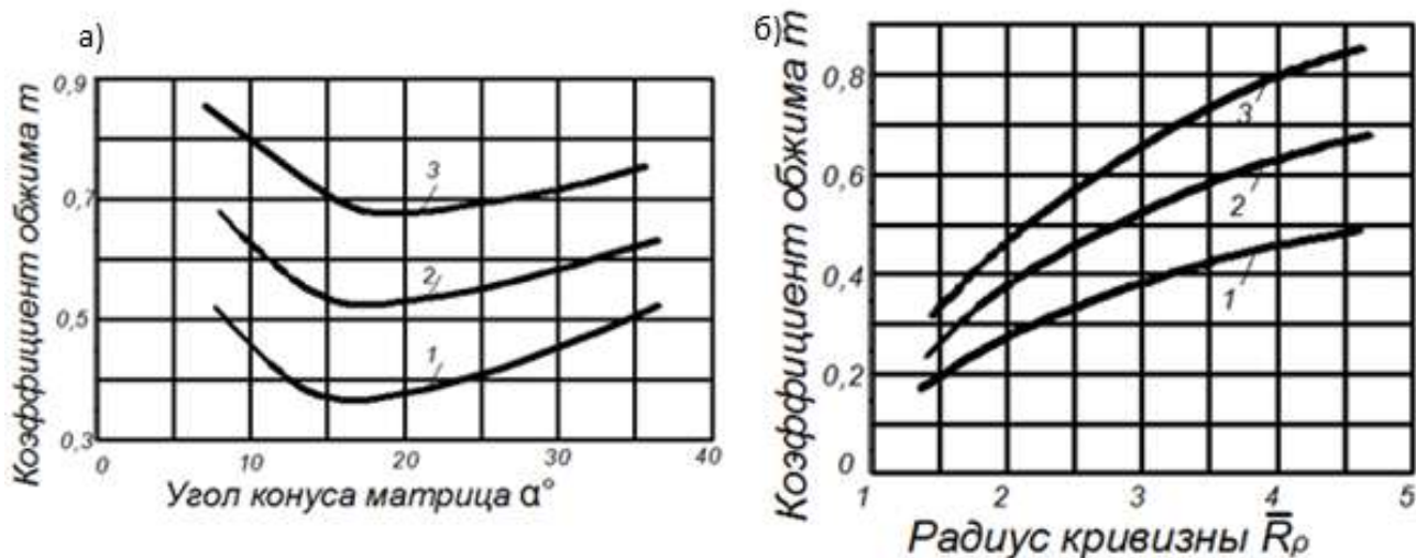
Рис. 4. Изменение предельного коэффициента обжима в зависимости: а) от угла конусности матрицы \alpha : 1 – n = 0,1 ; 2 – n = 0,3 ; 3 – n = 0,5 . б) от радиуса кривизны матрицы R_{ск} : 1 – n = 0,1 ; 2 – n = 0,3 ; 3 – n = 0,5 .
