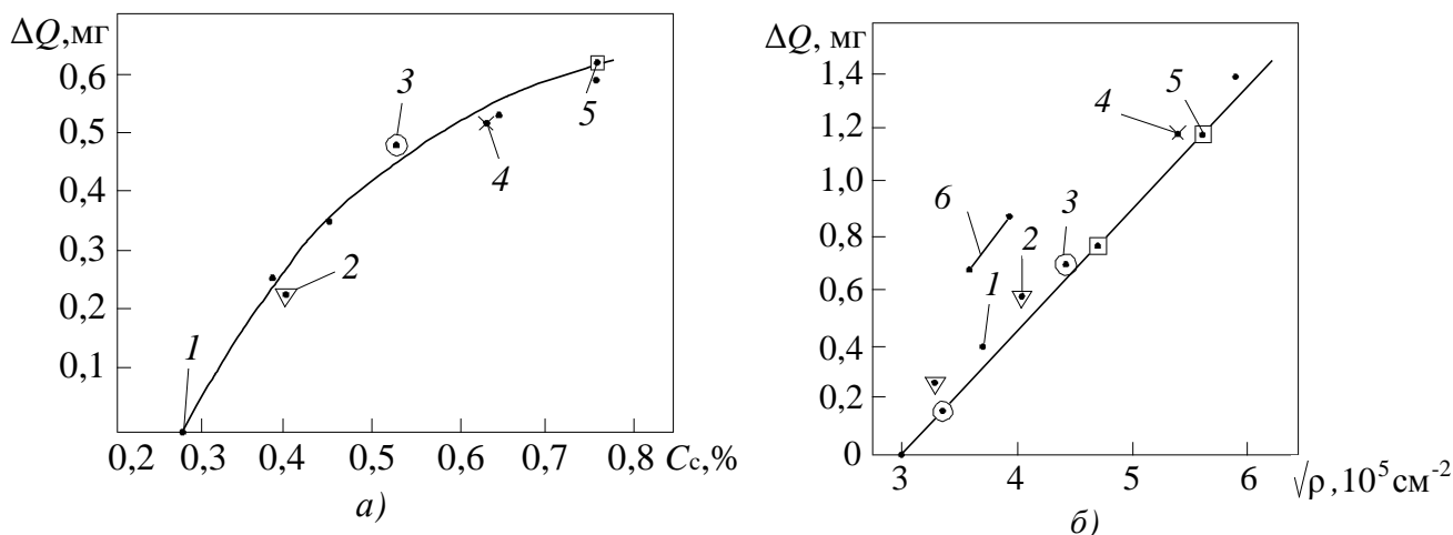
Рисунок 2. Значения разниц \Delta Q износ для сталей 30 (1), 45 (2), 55 (3), 65Г (4), У8 (5) и стали 30 без отпуска (6) в зависимости от содержания C_C углерода в мартенсите (а) и от плотности \sqrt{\rho} дислокаций (б), а также их аппроксимирующие кривые
