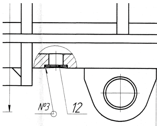
Рисунок 4 – Сварной шов №3
